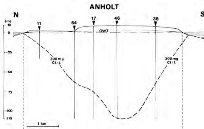
Figur 5. Tværsnit gennem Ørkenen (for placering se figur 4), visende grundvandet højde (GWT) og tykkelsen af ferskvands-puden. Der er en overgangzone mellem det ferske og det salte grundvand. Her er vist beliggenheden af den dybde, hvor klorid indholdet når 300 mg/l.
