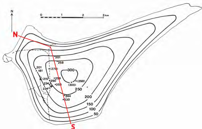
Figur 4. Grundvandshøjden over havniveau – i cm – observeret 1973 i forbindelse med undersøgelserne forud for etableringen af indvindingsboringerne i Ørkenen. N-S profilet er vist i figur 5.
