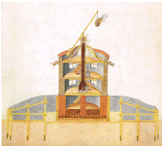
Forslag i 1701 til opførelse af et tårn med vippefyr på Anholt Knob
